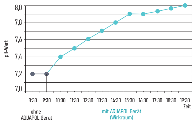
Messung des pH-Wertes im Leitungswasser ohne/mit AQUAPOL Entfeuchtungssystem (Wirkraum)
